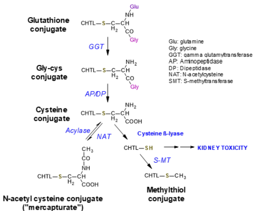
Figure 3 : Mécanisme de bioactivation du chlorothalonil (EFSA, 2017b)
